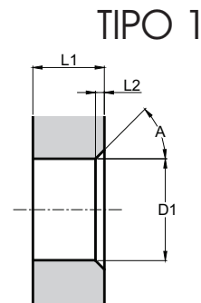
Ferramenta especial para furar e chanfrar
