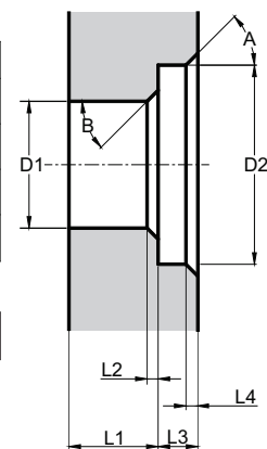
Ferramenta especial para furar, chanfrar, facear e chanfrar
